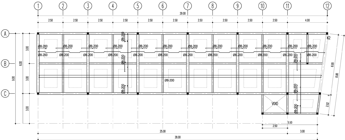
RENCANA PENULANGAN PLAT LANTAI 2 Skala 1 : 150
