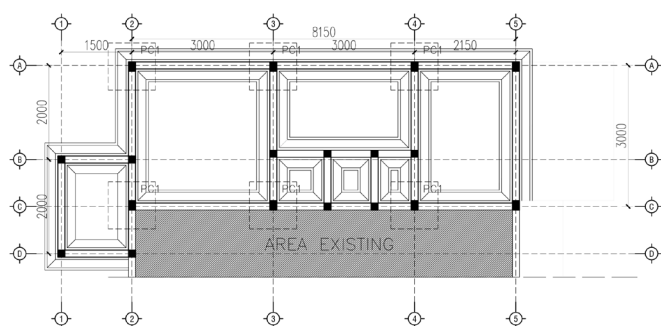
RENCANA PONDASI SKALA 1:100
