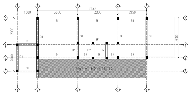
RENCANA BALOK SKALA 1:100
