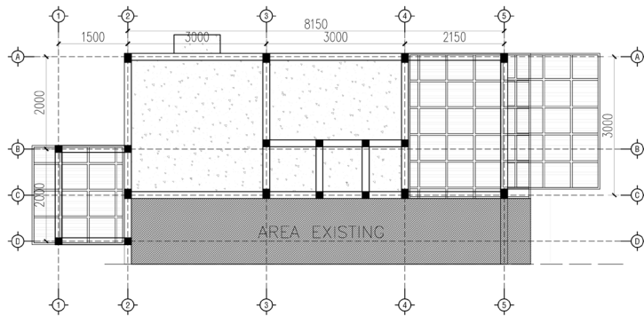
RENCANA ATAP SKALA 1:100
