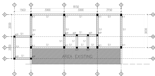
RENCANA KOLOM DAN SLOOF SKALA 1:100
