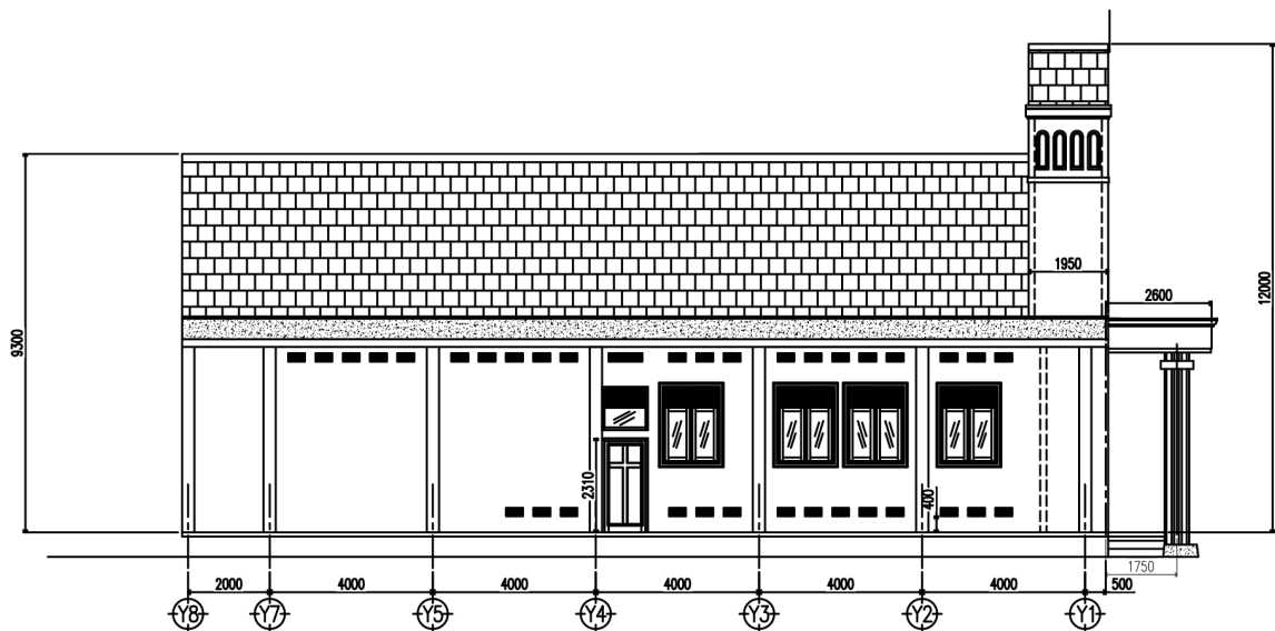
TAMPAK SAMPING [PANDANGAN UTARA]
