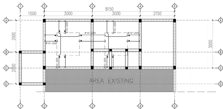
PENULANGAN PLAT ATAP SKALA 1:100
